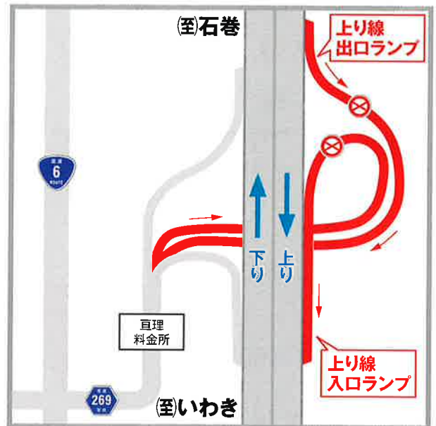
亘理IC 上り線出入口ランプ閉鎖図
